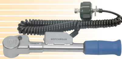
締付トルクの上下限管理が可能な 空転式トルクレンチの例 QSPCAMS
