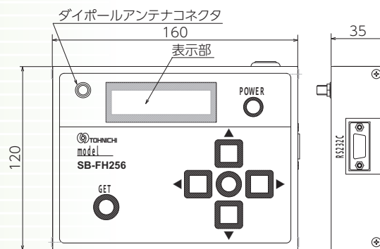
設定ボックス SB-FH256
