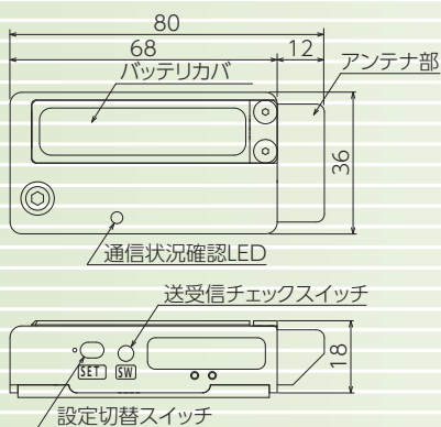
送信機 T-FH256MC
