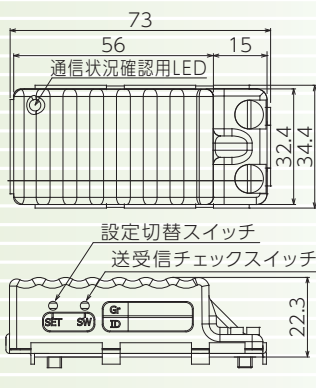
小型送信機 T-FHLS256
