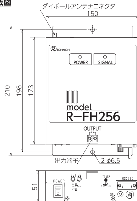
受信機 R-FH256
